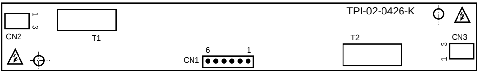
Рисунок 8.2 – Разъёмы платы конвертора TFT типа TPI-02-0426-K
