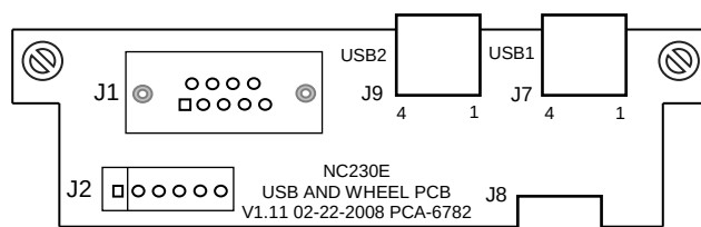
Рисунок А.4 - Расположение разъемов платы NC210-27
