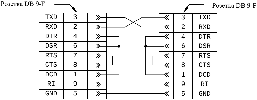
а) минимальный кабель RS-232
